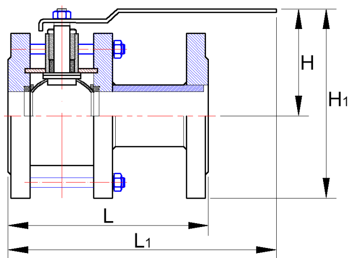
Рисунок 2. Размеры крана 11с41фт
