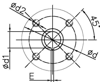
Присоединительный фланец
